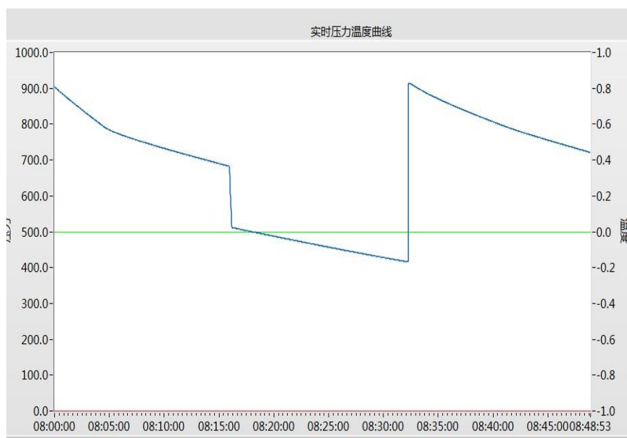
图 1 压力相关法原理图
