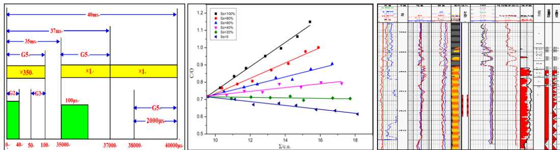
双循环脉冲发射模式及双参数测井响应
