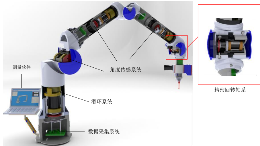
图 1 测量机外观示意图
