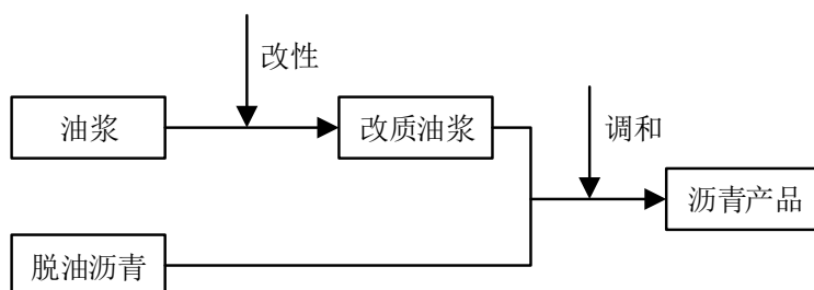
图 1 催化油浆改性制备石油沥青工艺
