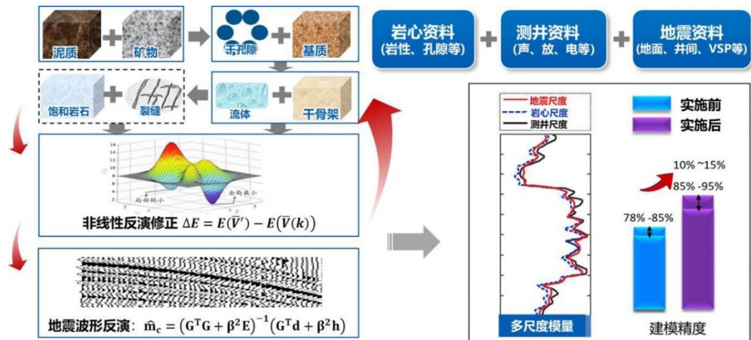
图1 多元多尺度迭代岩石物理建模
