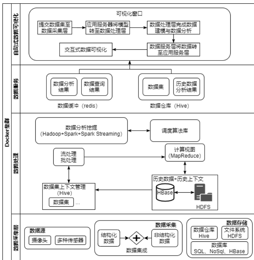
图 3 系统架构图
