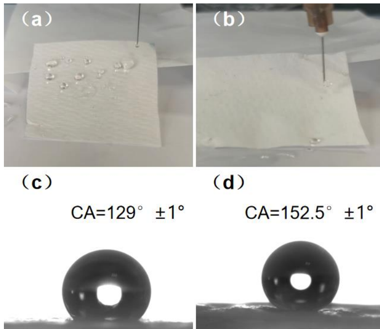
图 3 超疏水改性前后的聚丙烯熔喷布对水滴的润湿性对比
