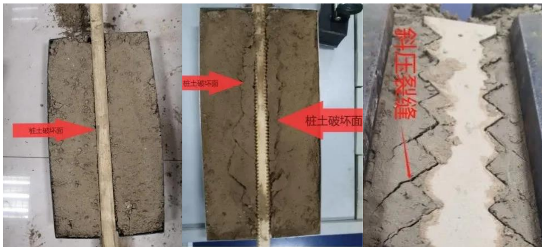
图 2 侧压增强桩实验
