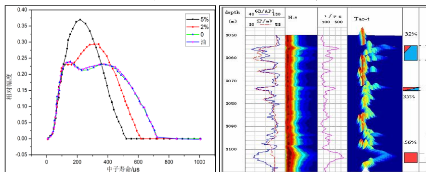
不同地层条件中子寿命分布及热中子成像油气指示
