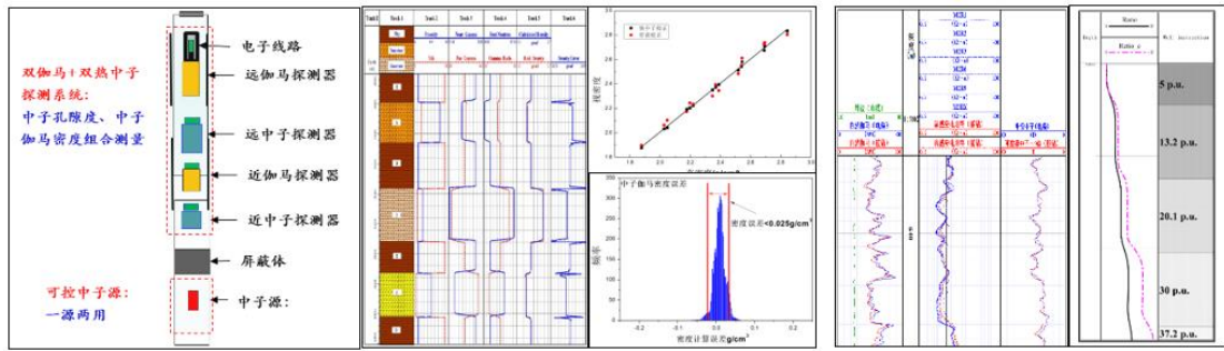
可控中子源中子密度组合测量方法及结果对比
