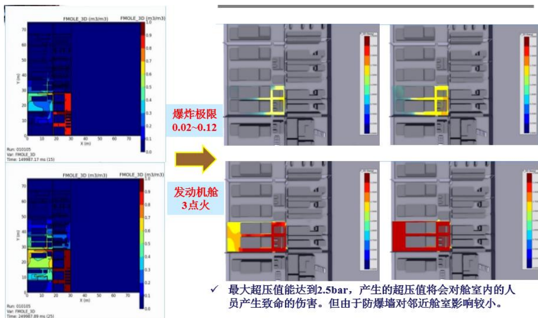
图2 隐患排查模拟功能模块
