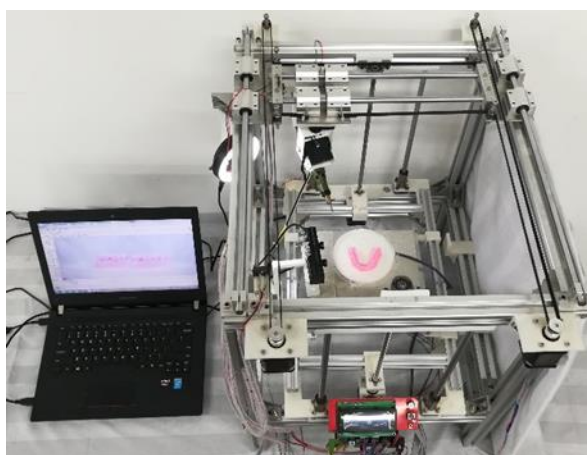
图 6 切割试验平台整体实物图
