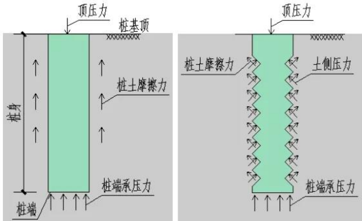
图 1 侧压增强桩技术原理示意图
