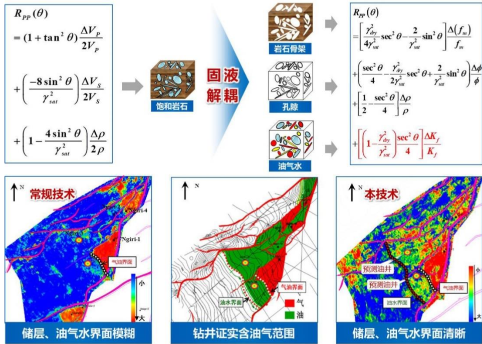
图 3 固液解耦地震油气识别
