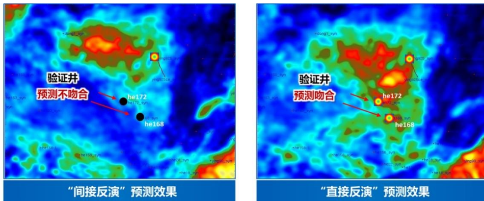
图2 多类型复杂储层特征参数叠前地震直接反演
