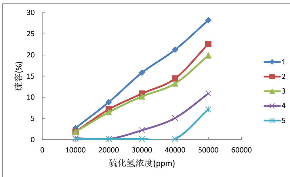
图 2 硫化氢浓度对硫容的影响
