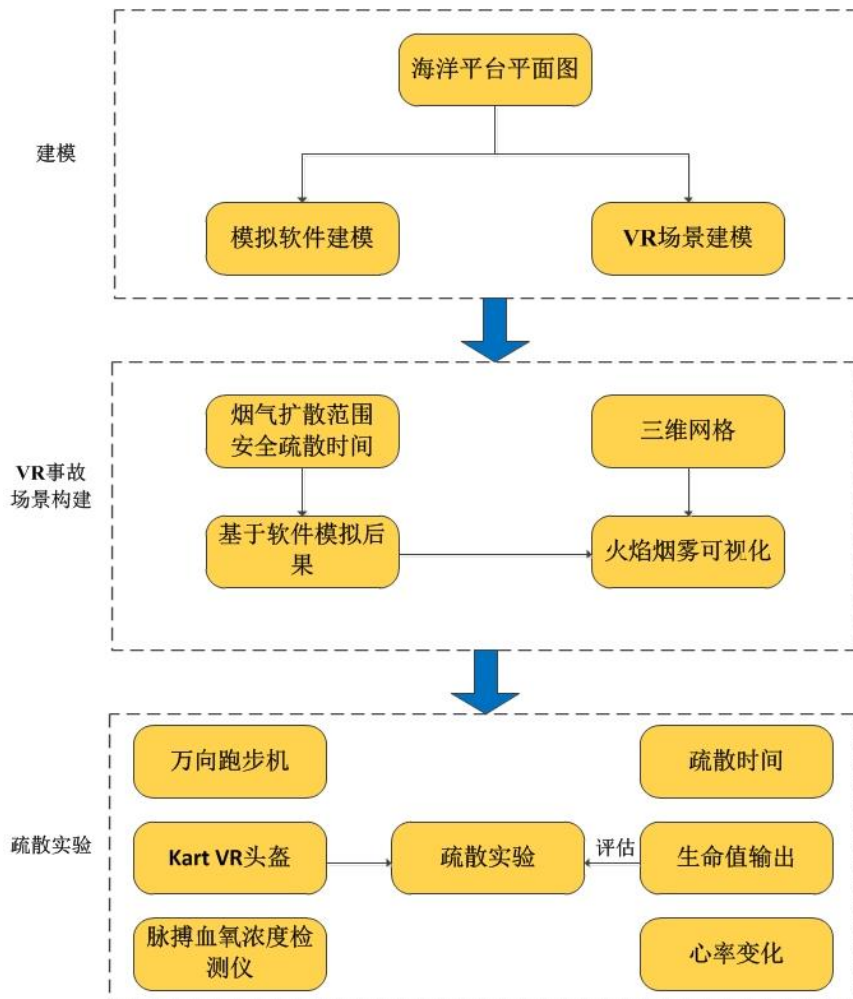
图3 火灾爆炸后果影响嵌入 VR 原理流程图
