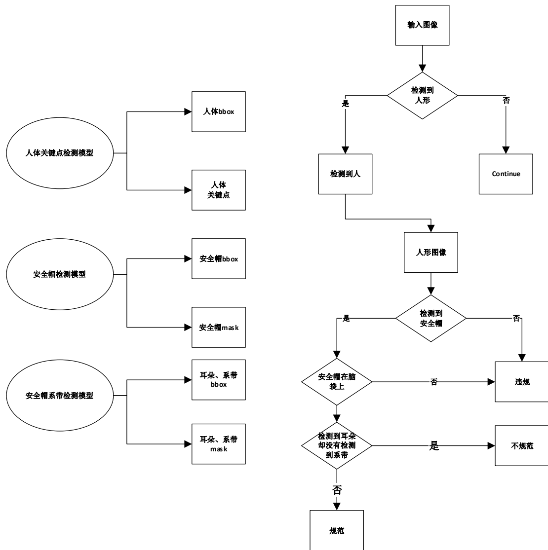
图 3 安全帽佩戴规范检测
