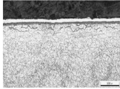
图 2 渗氮层横截面组织特征
