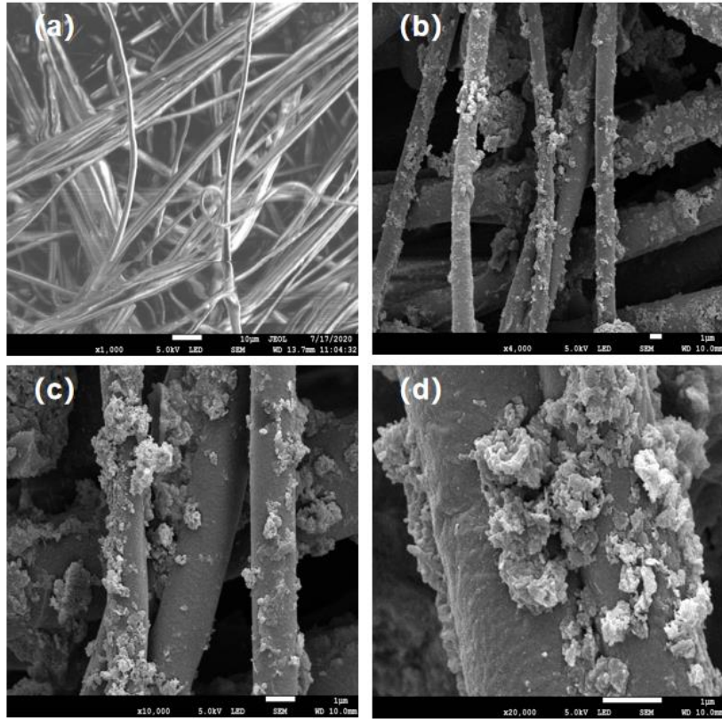
图 2 SEM 图 (a): 原始聚丙烯熔喷布; (b), (c), (d): 经过喷涂改性后的聚丙烯熔喷布。
