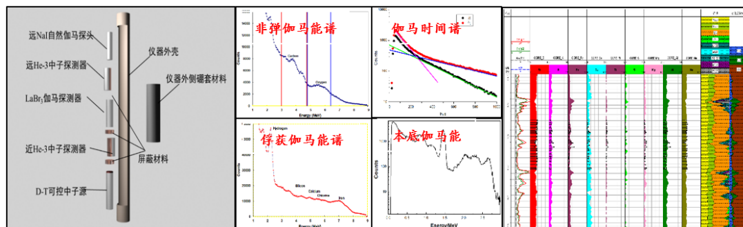
多探测元素测量方法及结果对比
