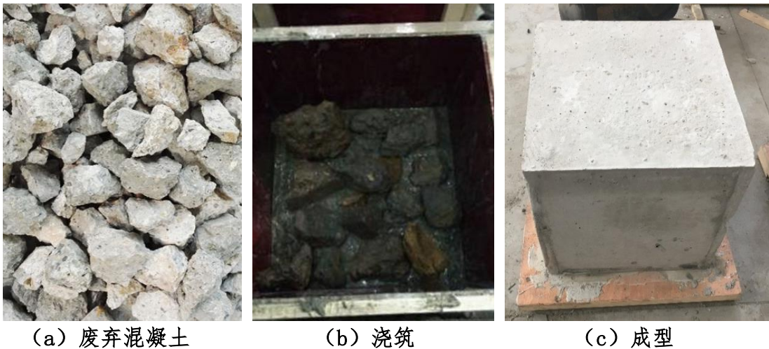
图 1 再生大骨料自密实混凝土制备过程
