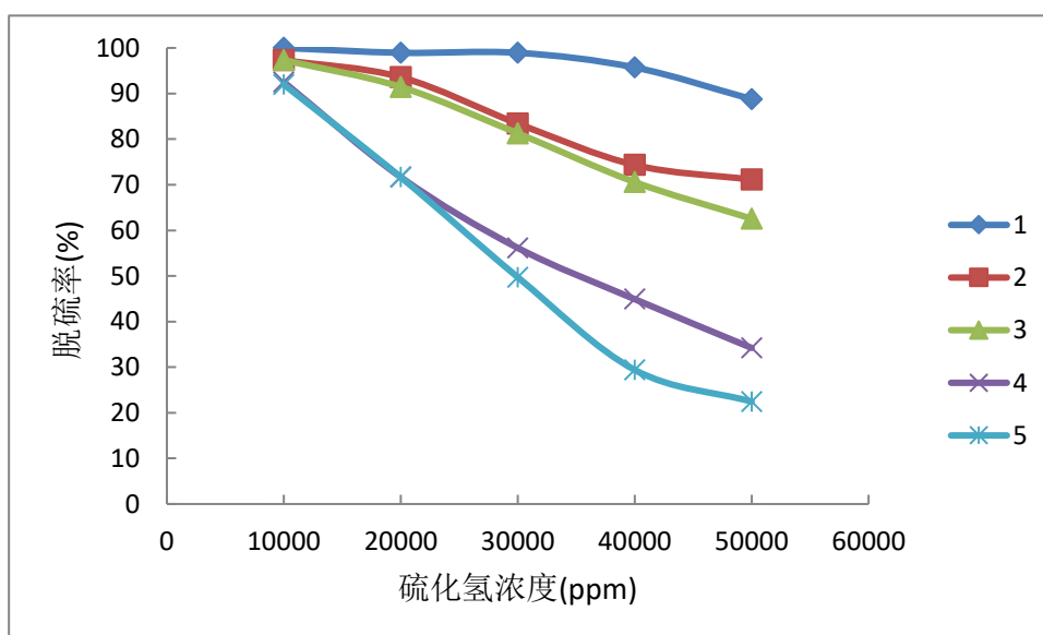
图 3 硫化氢浓度对脱硫率的影响
