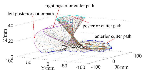
图 2 刀具路径示意图
