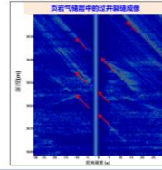
页岩气储层中的过井裂隙成像
