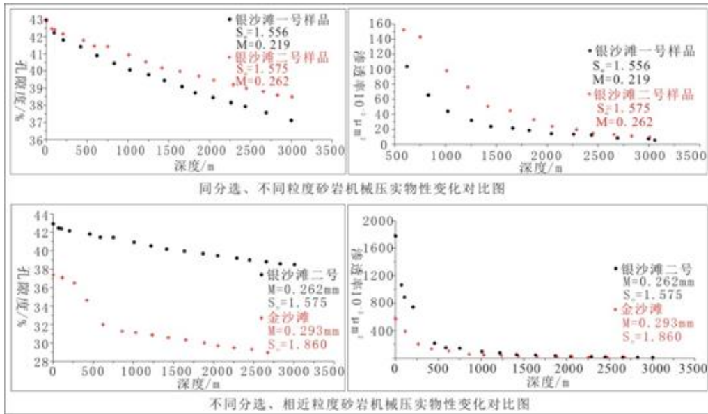
粒度和分选对砂岩机械压实作用的影响
